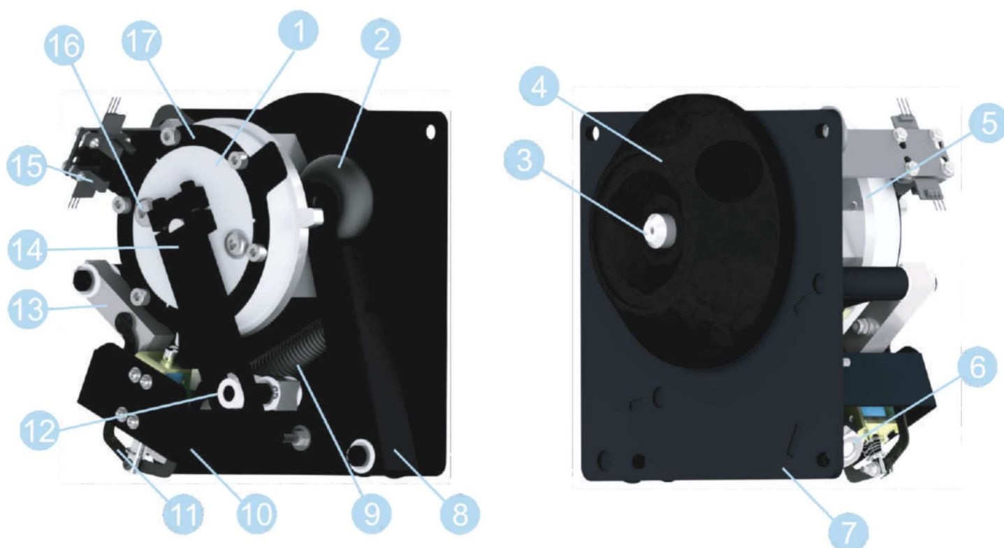
Рисунок 12.2.1 - Расположение узлов механизма турникета TM-1
