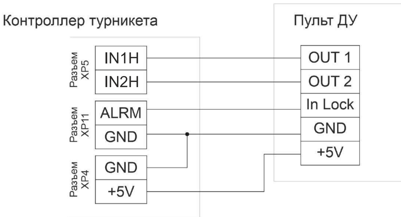
Рисунок 8.1.1 - Подключение ПДУ к турникету
