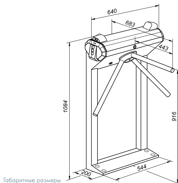
Габаритные размеры
