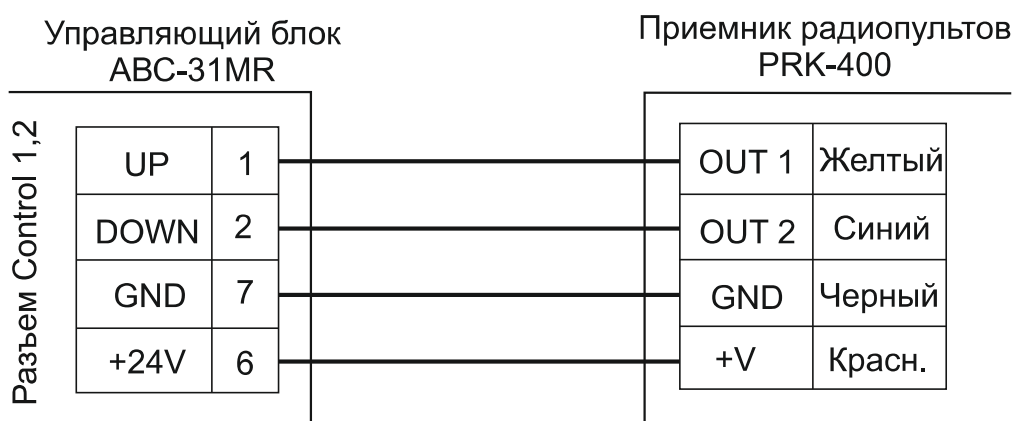
Рисунок 6.6.4. Схема подключения приемника радиопультов
