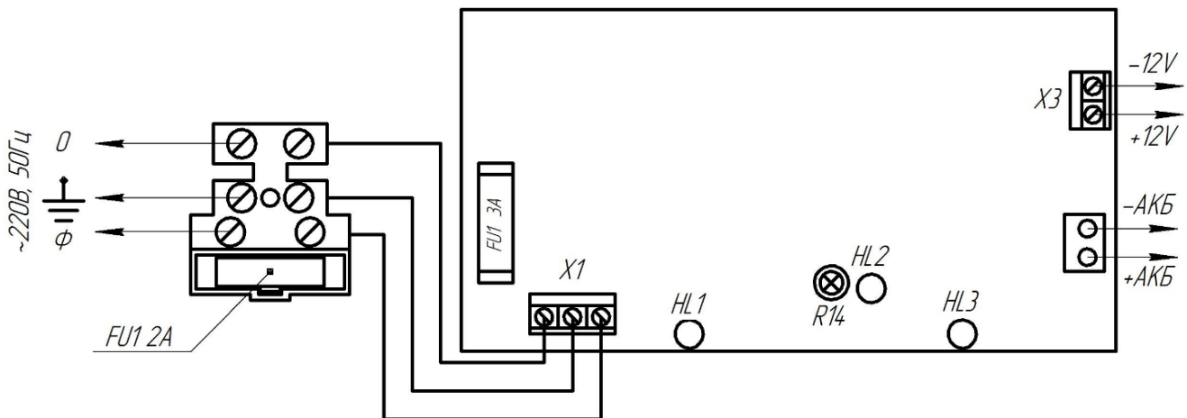
Рис. 1 Схема подключения
