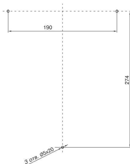
Схема разметки отверстий для блока управления
