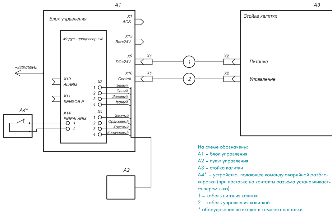
Схема электрических соединений калитки PERCO-WMD-05S
